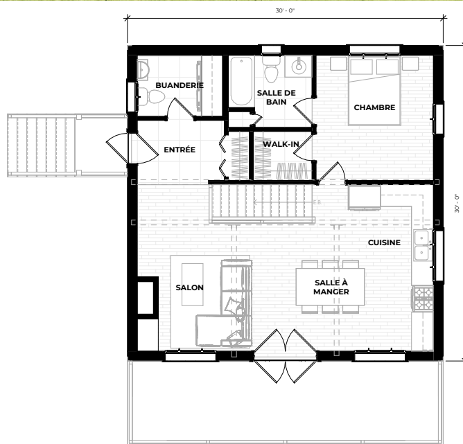
REZ-DE-CHAUSSÉE
