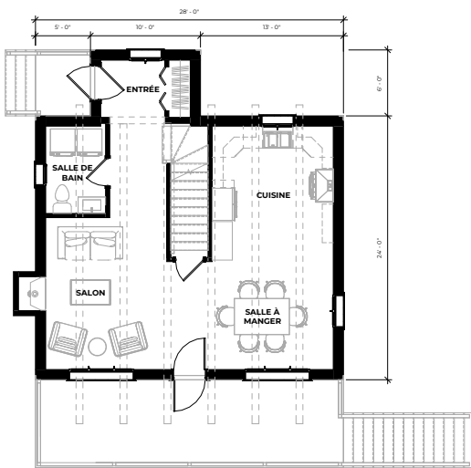
REZ-DE-CHAUSSÉE
